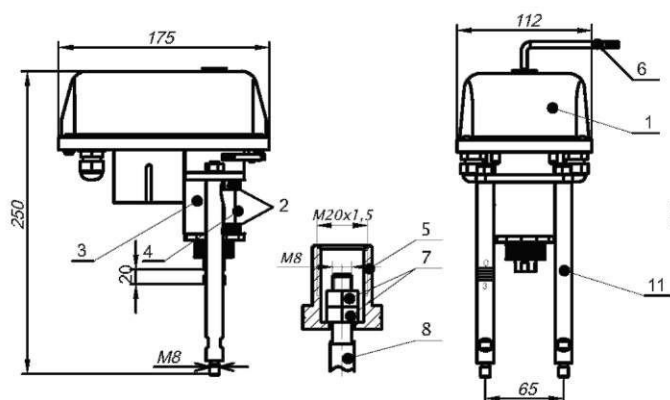
Рисунок 1. ВЭП-05-3000, ВЭП-15-3000, ВЭП-25-3000
