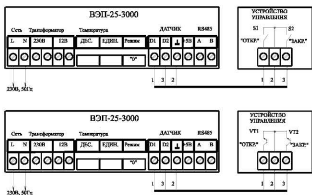
Рисунок 13. Схемы подключения ВЭП-2Х-3000 при работе в режиме "0"
