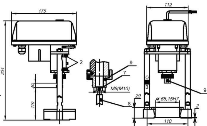
Рисунок 2. ВЭП-06-3000, ВЭП-16-3000, ВЭП-26-3000
