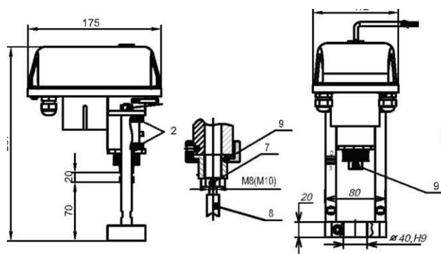
Рисунок 3. ВЭП-07-3000, ВЭП-17-3000, ВЭП-27-3000
