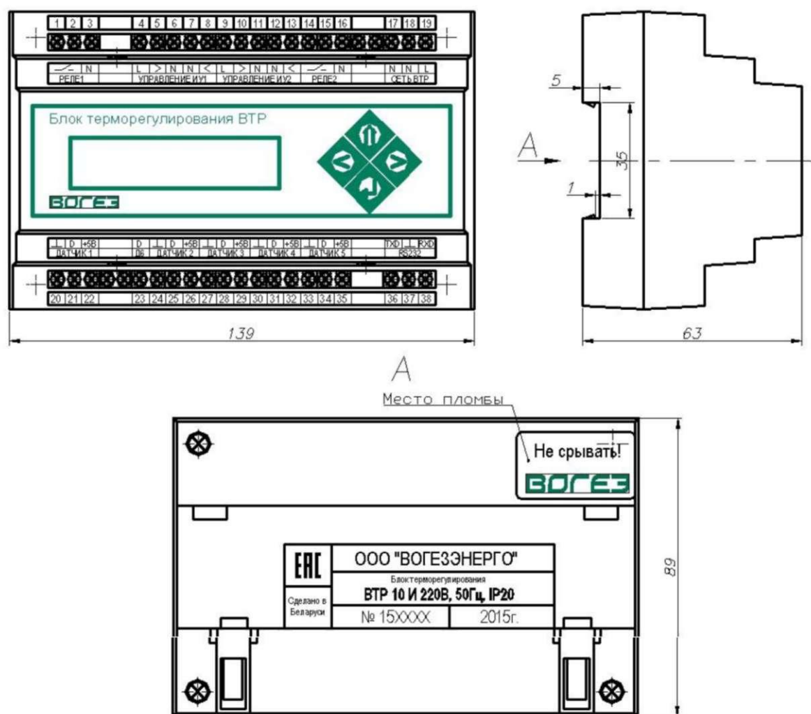
Рисунок А.1 Габаритные и установочные размеры блока терморегулирования ВТР-10И
