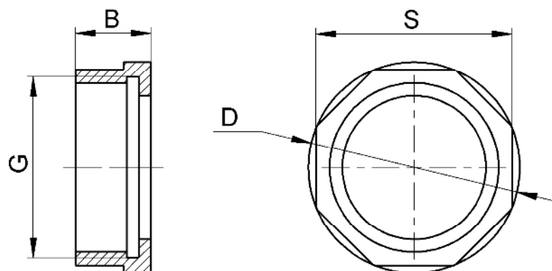
Гайка
