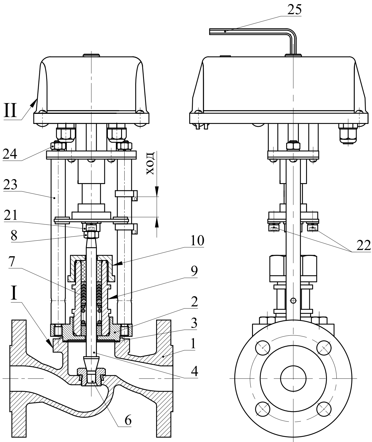
Рисунок 1 - DN15, Kvy 0,25; 0,4
